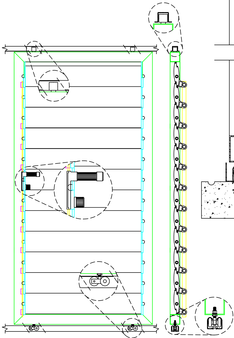
Alzado interior y sección de la persiana corredera dentro de hueco, con detalles de las fijaciones a fábrica Escala 1:8
