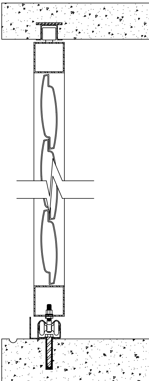
Sección constructiva de persiana corredera dentro de hueco. Escala 1:3
