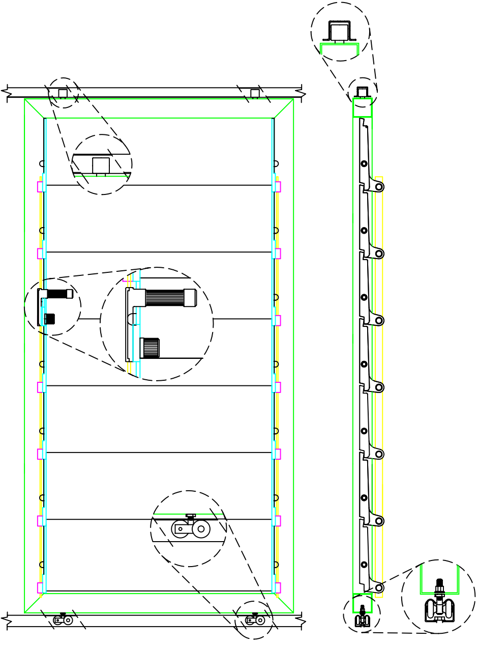
Alzado interior y sección de la persiana corredera dentro de hueco, con detalles de las fijaciones a fábrica. Escala 1:8
