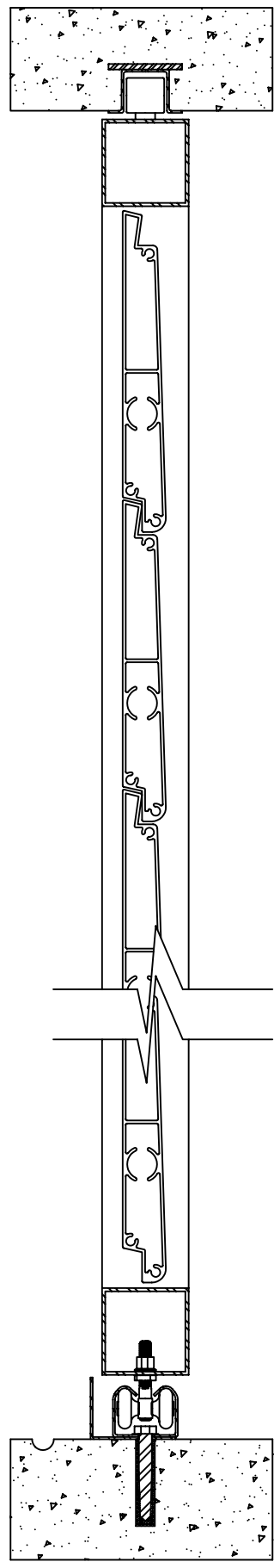
Sección constructiva de persiana corredera dentro de hueco. Escala 1:3
