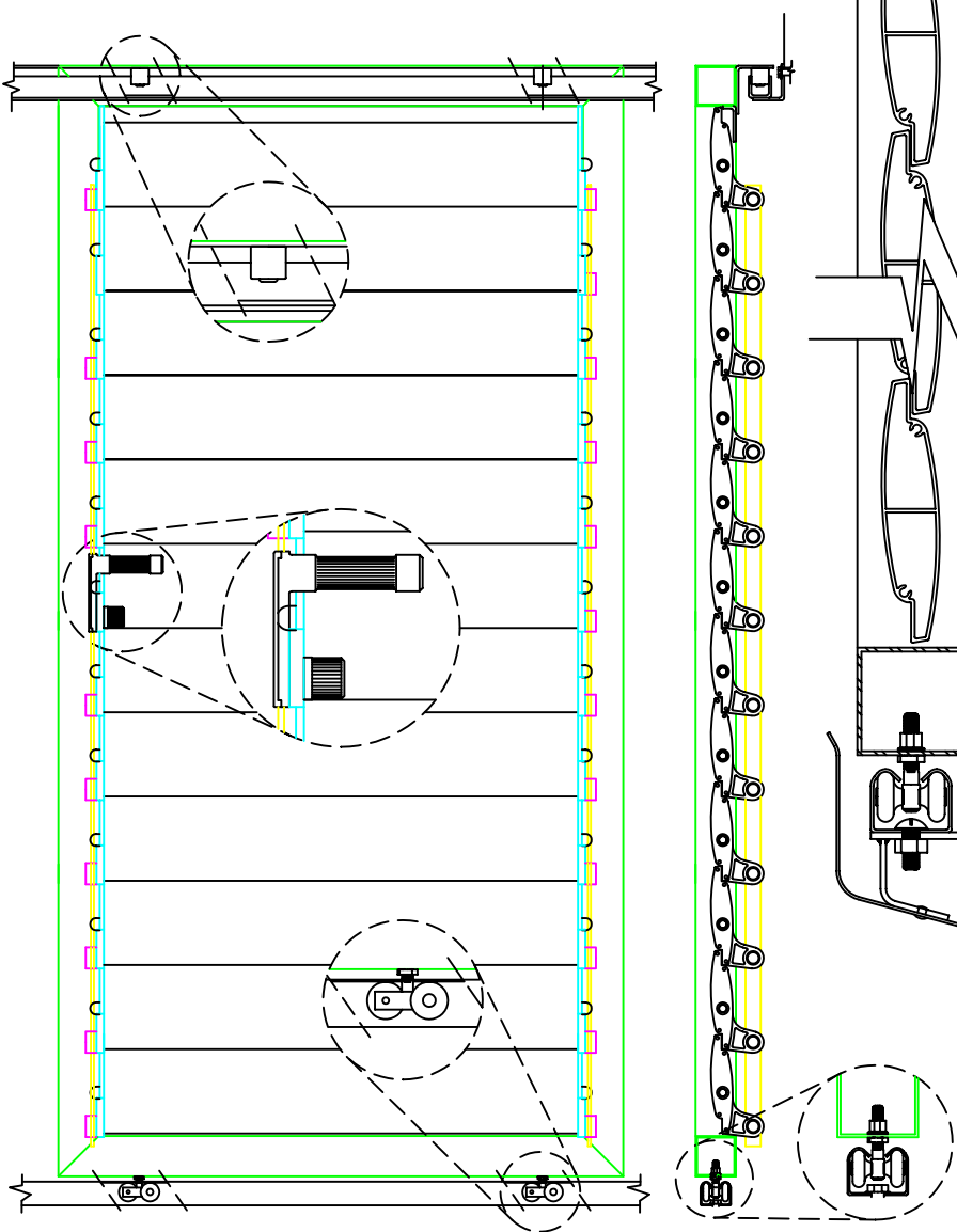
Alzado interior y sección de la persiana corredera en fachada, con detalles de las fijaciones a fábrica Escala 1:8
