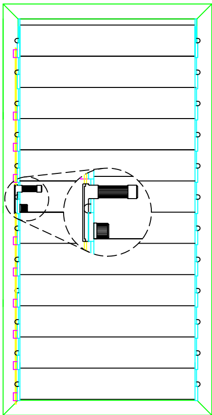
Alzado interior y perfil de la lama fija orientable. Escala 1:10
