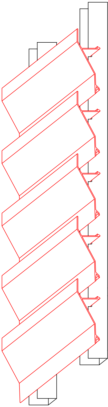
Detalle de Perspectiva de Celosía fija MY 100 AF Escala 1:3
