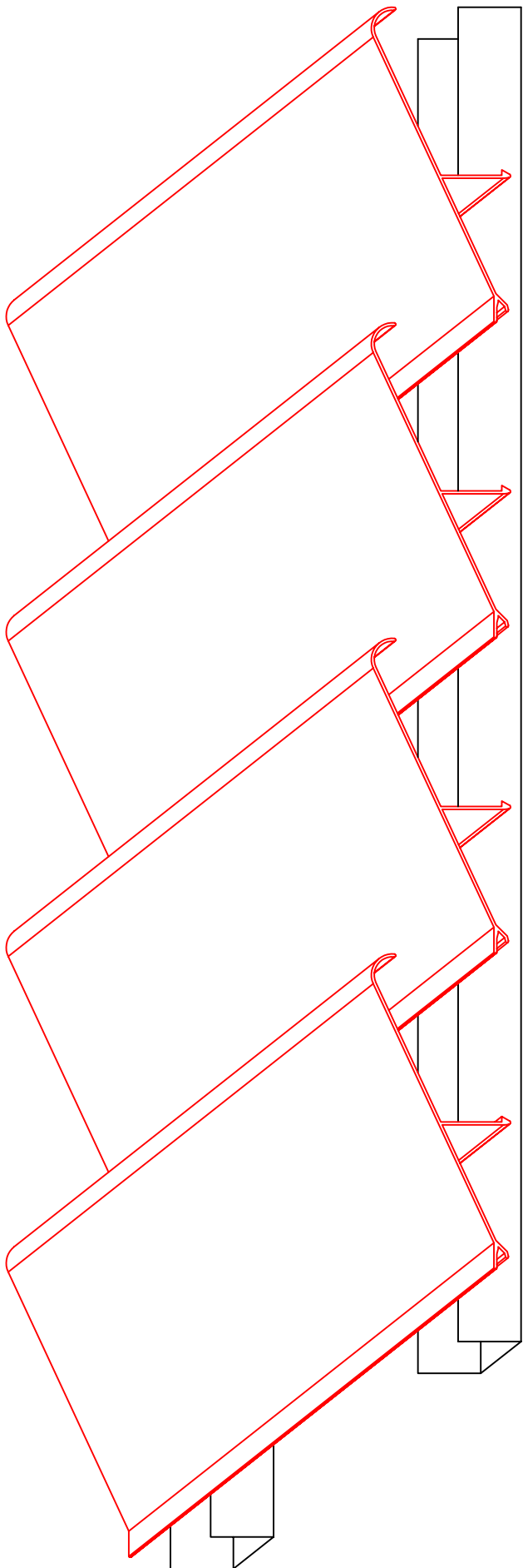
Detalle de Perspectiva de Celosía fija MY 150 AF Escala 1:3
