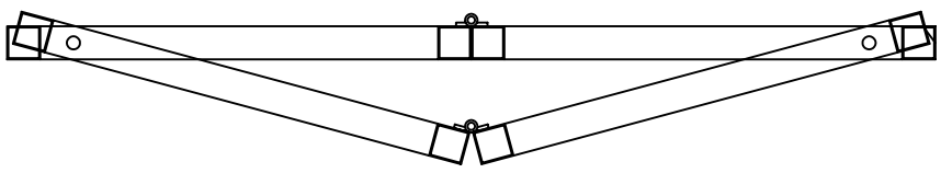
Alzado interior, sección y planta de la persiana plegable dentro de hueco. Escala 1:10
