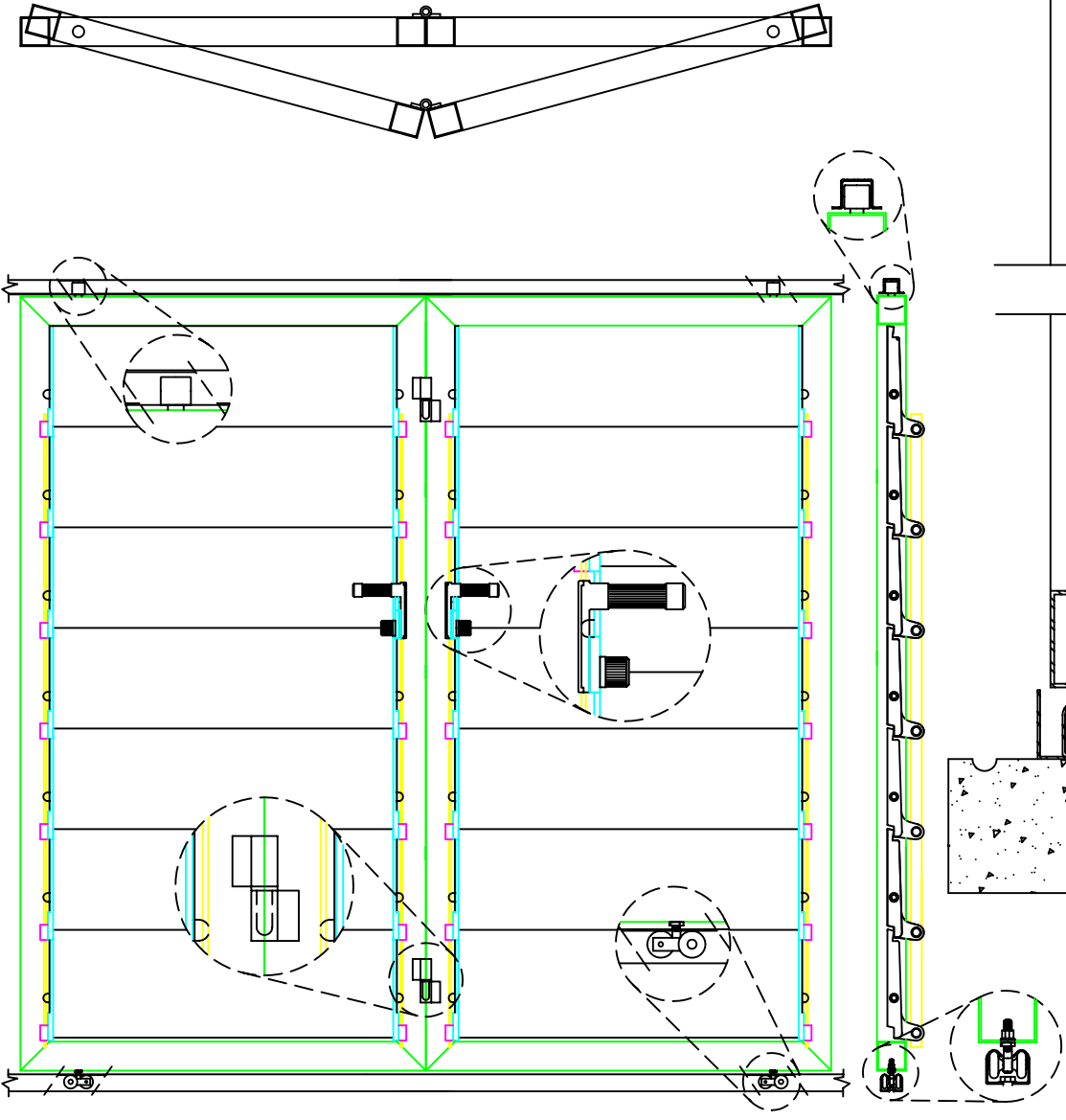
Alzado interior, sección y planta de la persiana plegable dentro de hueco. Escala 1:10
