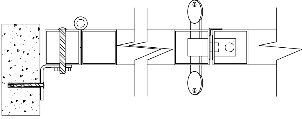
Sección detallada del sistema de apertura de la persiana practicable. Escala 1:2.5
