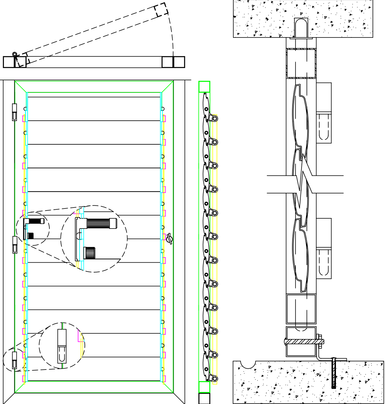
Sección constructiva de persiana practicable. Escala 1:3 Alzado interior, perfil y planta de persiana practicable. Escala 1:8
