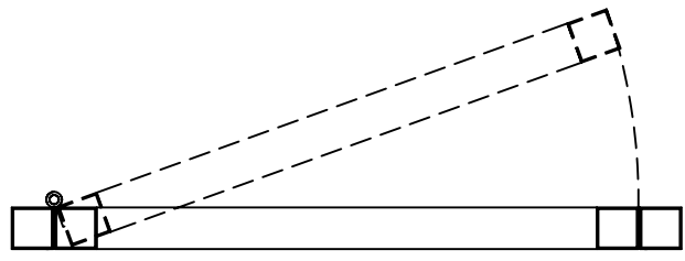
Sección constructiva de persiana practicable. Escala 1:3 Alzado interior, perfil y planta de persiana practicable. Escala 1:8
