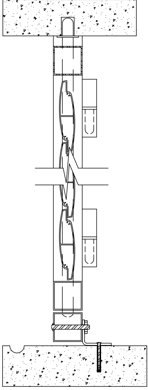
Sección constructiva de persiana practicable. Escala 1:3 Alzado interior, perfil y planta de persiana practicable. Escala 1:8
