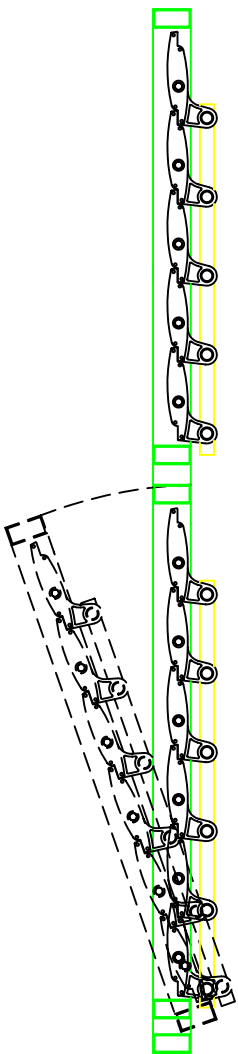
Alzado interior y perfil de la persiana proyectable con antepecho fijo. Escala 1:8
