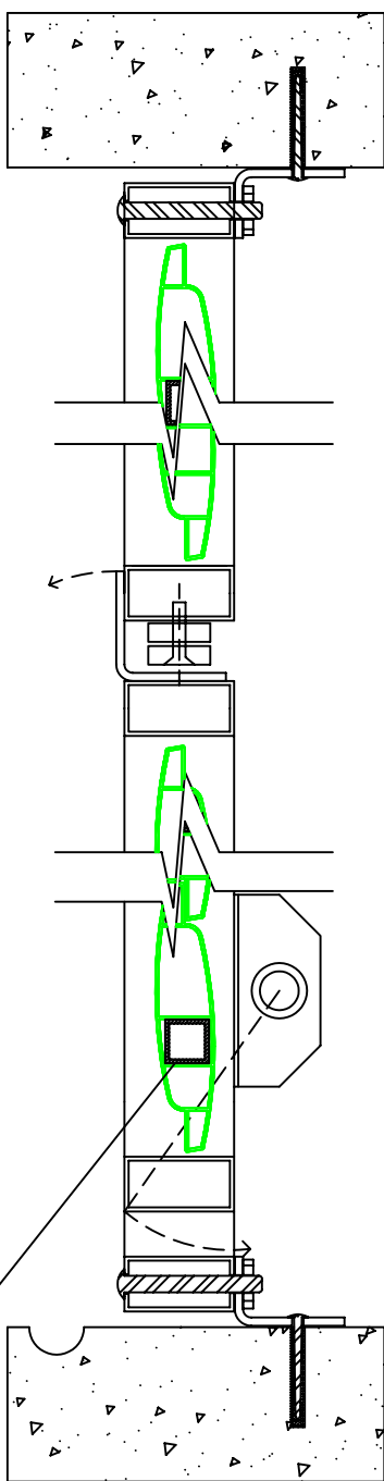
Sección constructiva de persiana proyectable con antepecho fijo. Escala 1:3
