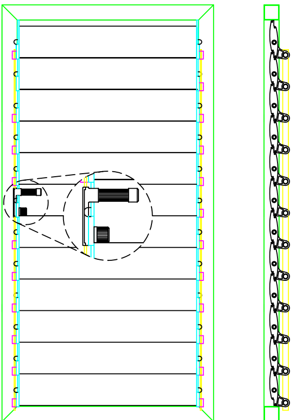
Alzado interior y perfil de la lama fija orientable. Escala 1:10
